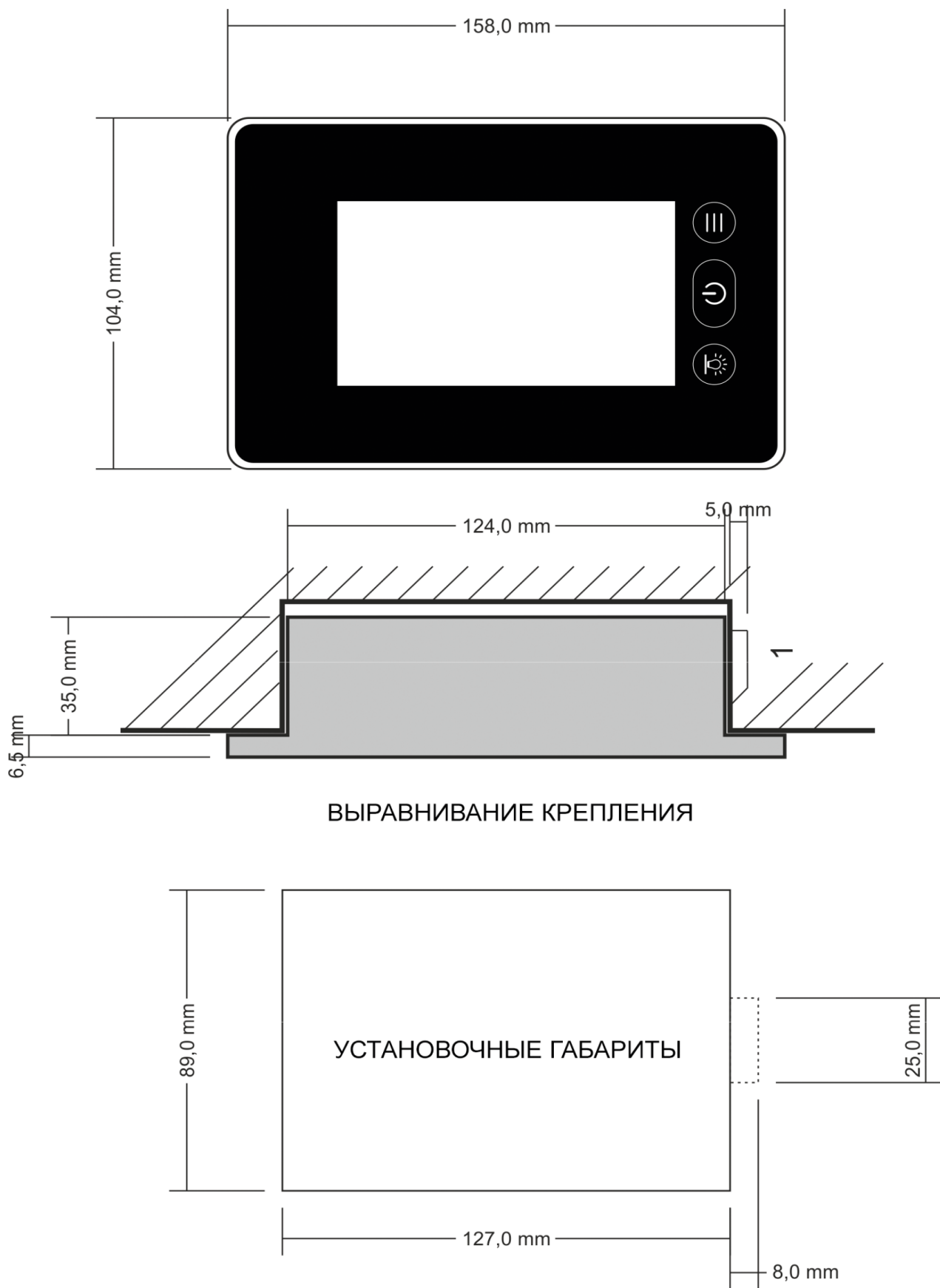
Рисунок 4. Установочные размеры
